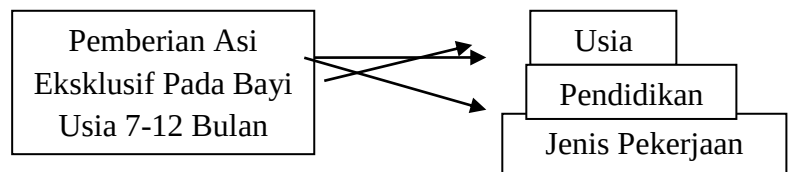
Gambar 3.1. Kerangka Konsep
